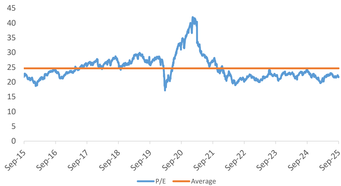
Nifty 50 P/E
